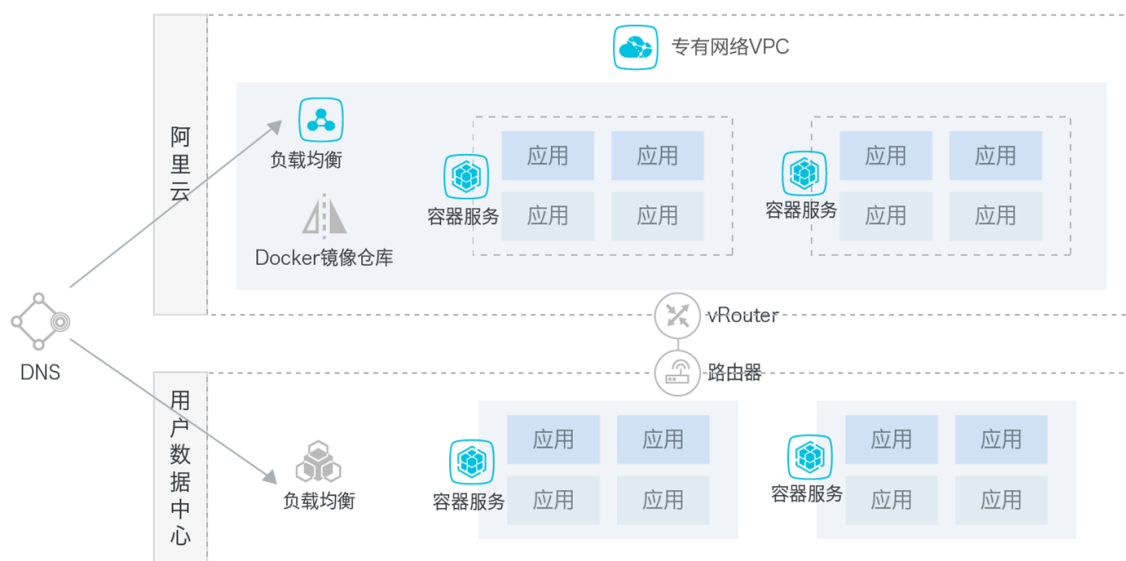
图 1-2: 架构方案
