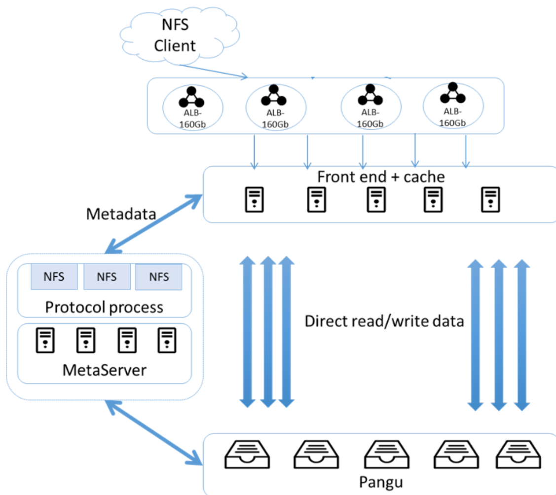
图 5-1: 系统架构图
