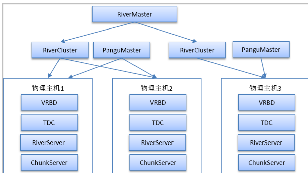
图 3-1: EBS软件架构
