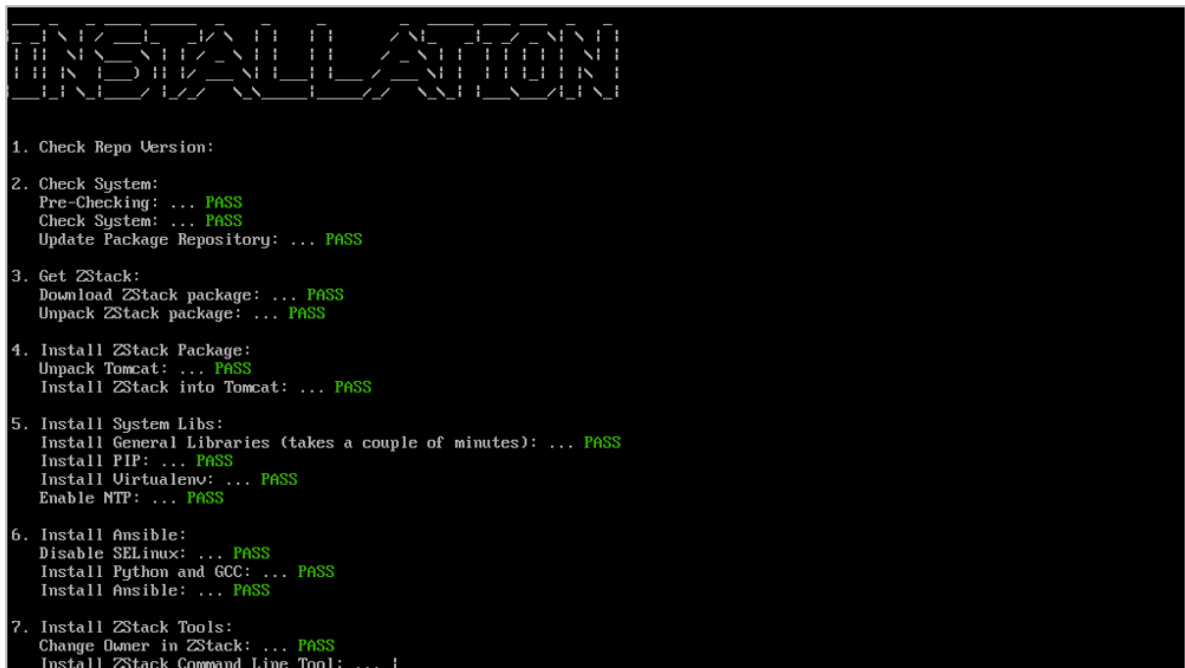
图 3-13: 自动安装管理节点
