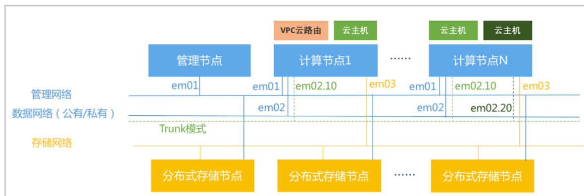
图 4-4: Ceph + VPC网络
