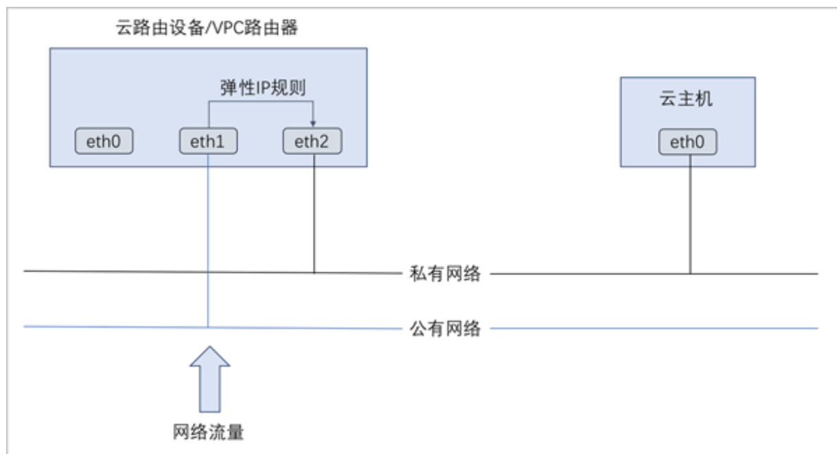
图 12-4: 云路由网络/VPC下弹性IP的应用场景
