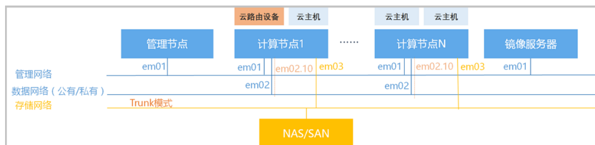
图 4-2: NAS/SAN +云路由网络
