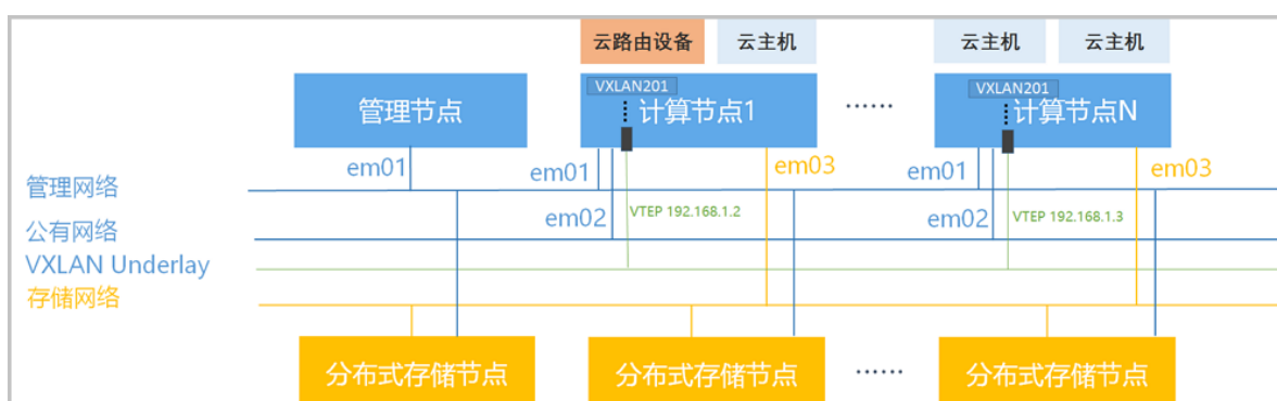
图 4-3: Ceph + VXLAN云路由网络
