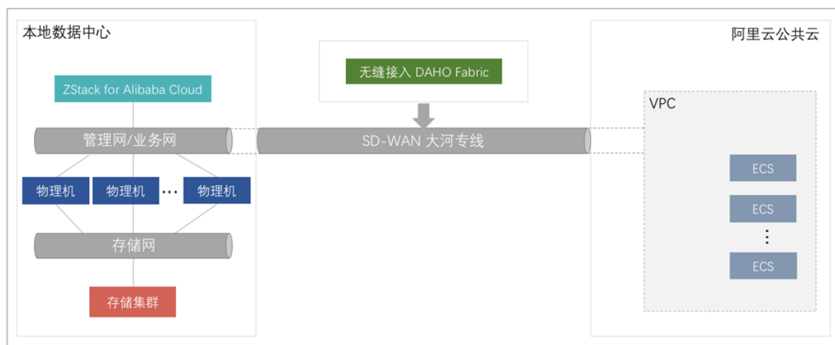
图 3-4: 基于SD-WAN部署
