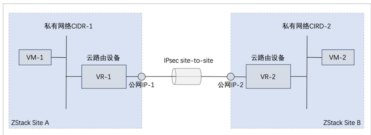
图 12-8: 云路由网络下IPsec隧道应用场景
