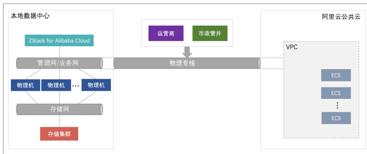
图 3-3: 基于物理专线部署
