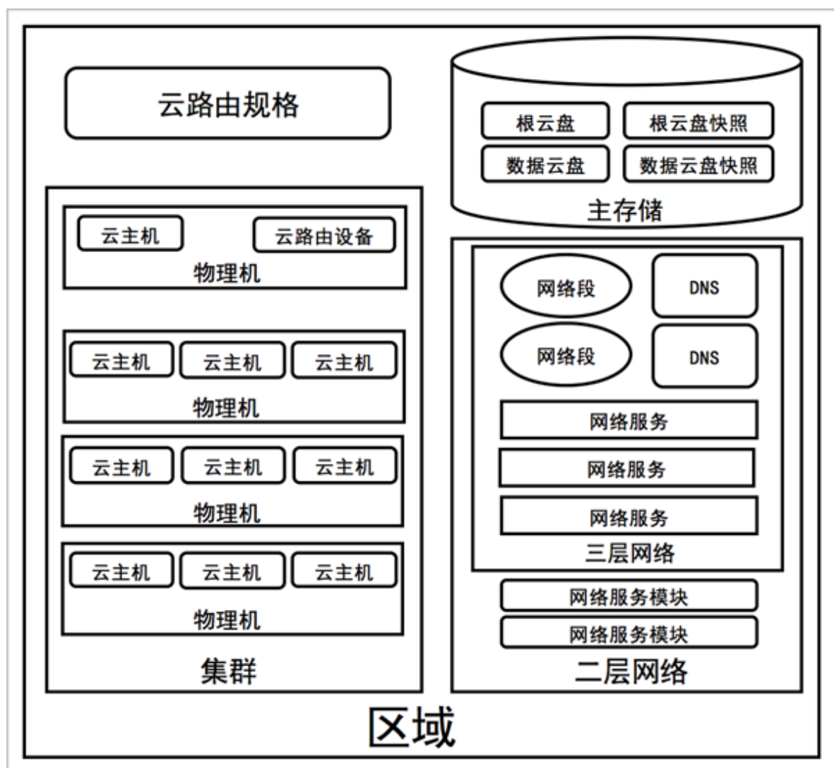
图 10-1: 区域资源结构
