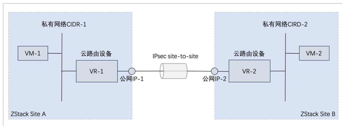
图 12-8: 云路由网络下IPsec隧道应用场景
