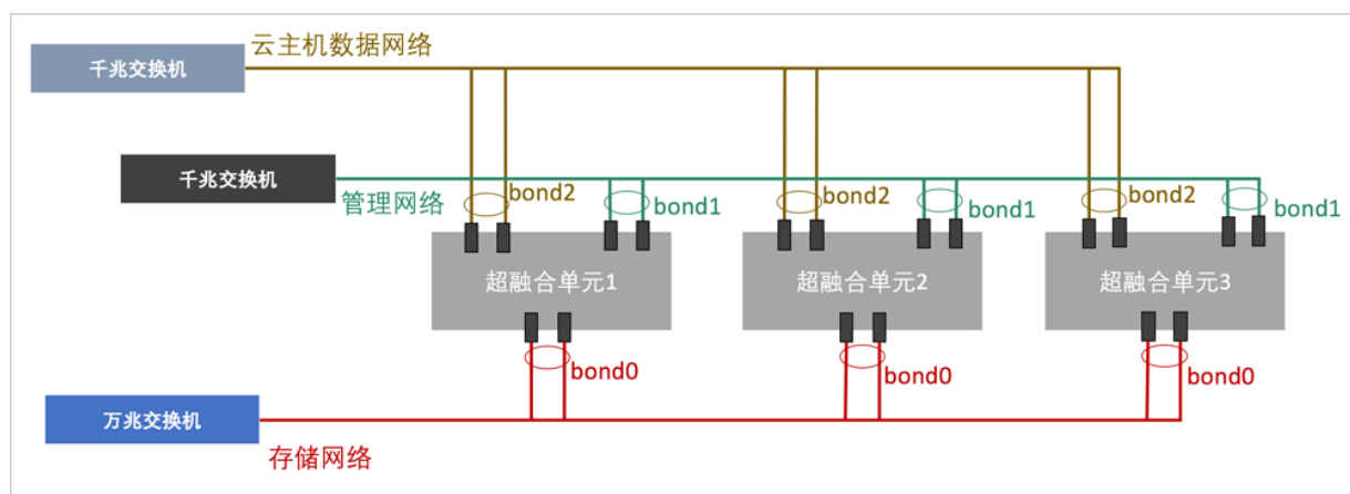
图 3: 超融合-三节点网络拓扑
