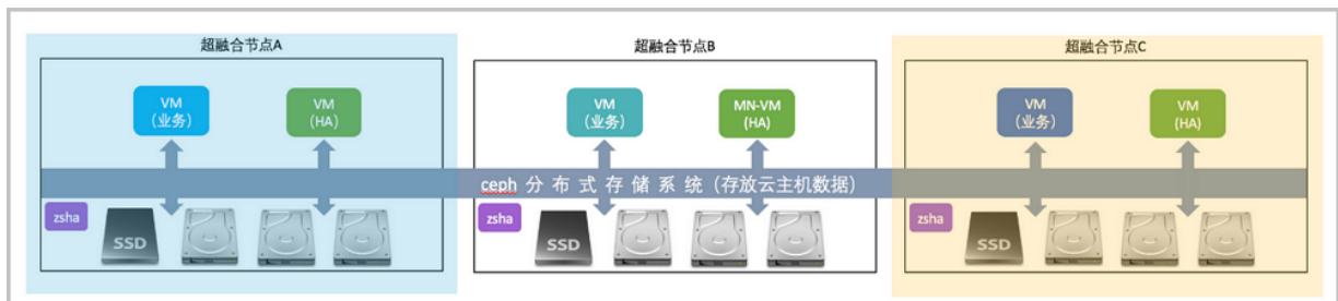
图 11: 超融合节点示例图
