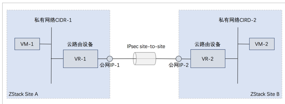
图 101: 云路由网络下IPsec隧道应用场景
