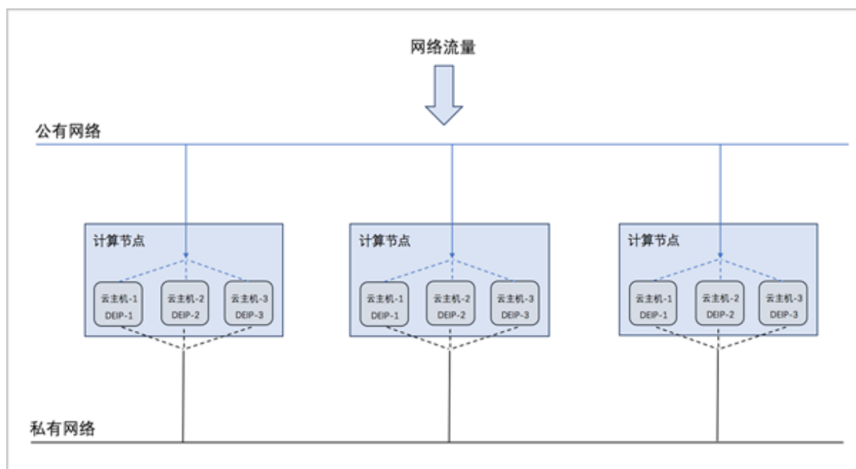
图 96: 扁平网络下弹性IP的应用场景
