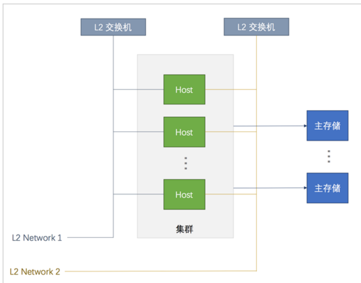
图 6: 集群、主存储、二层网络的关系
