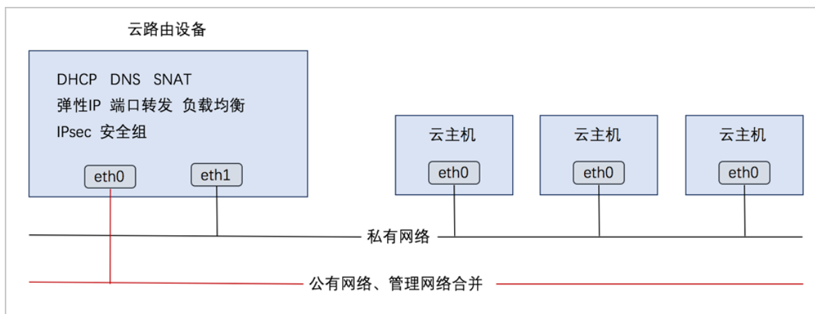
图 13: 部署方式-1
