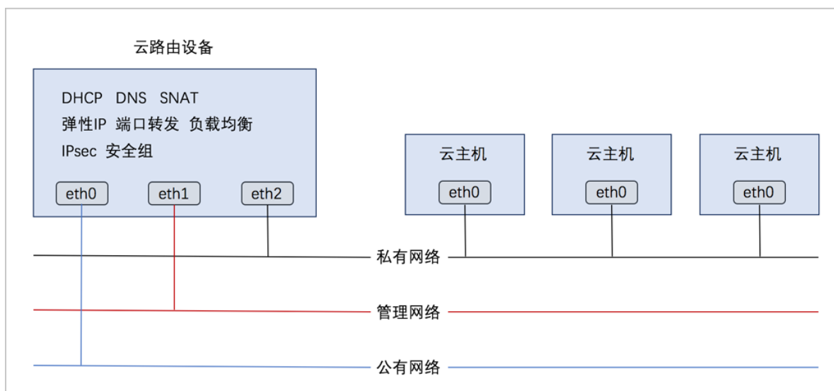
图 14: 部署方式-2
