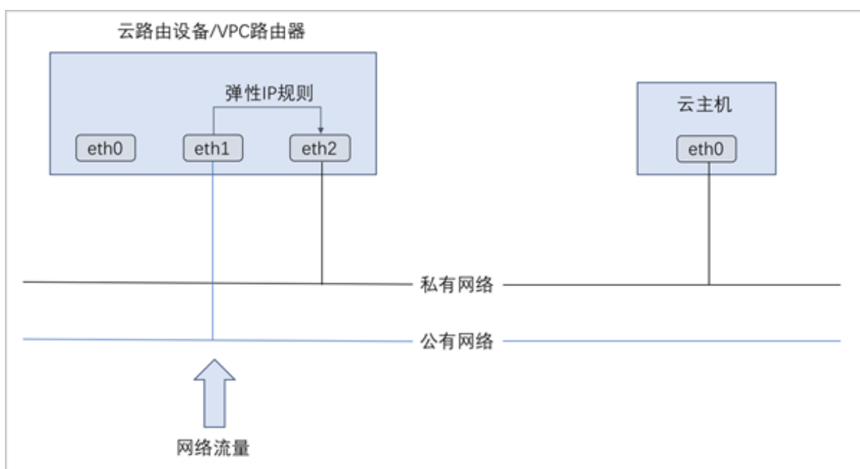
图 90: 云路由网络/VPC下弹性IP的应用场景
