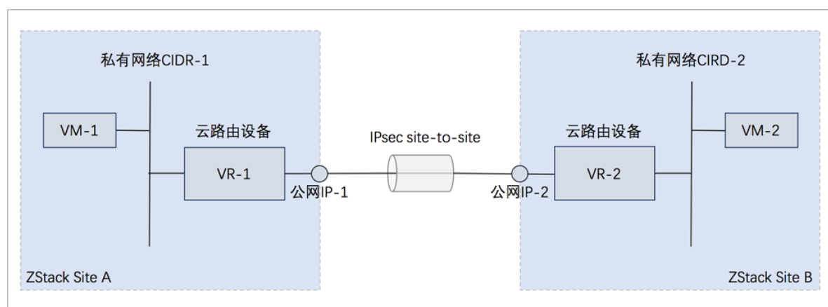
图 94: 云路由网络下IPsec隧道应用场景
