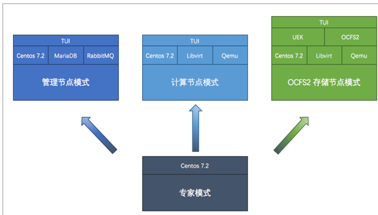
图 35: 四种安装模式示意图
