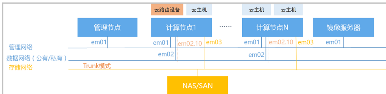
图 10: NAS/SAN +云路由网络
