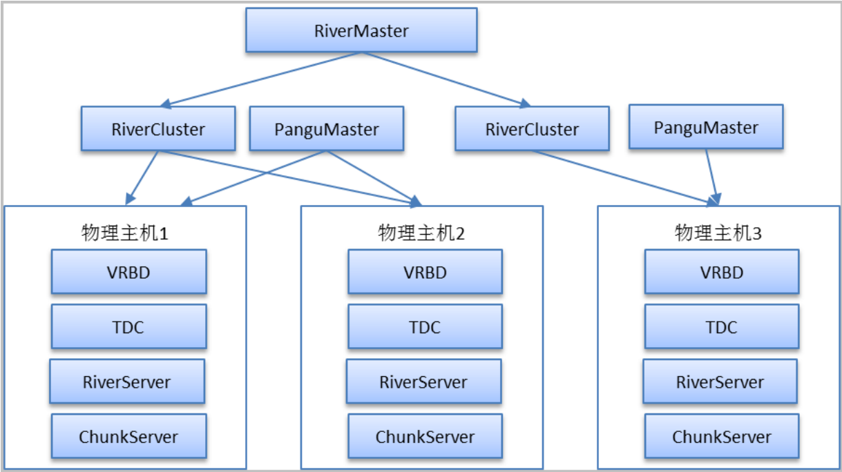
图 5-5: EBS软件架构
