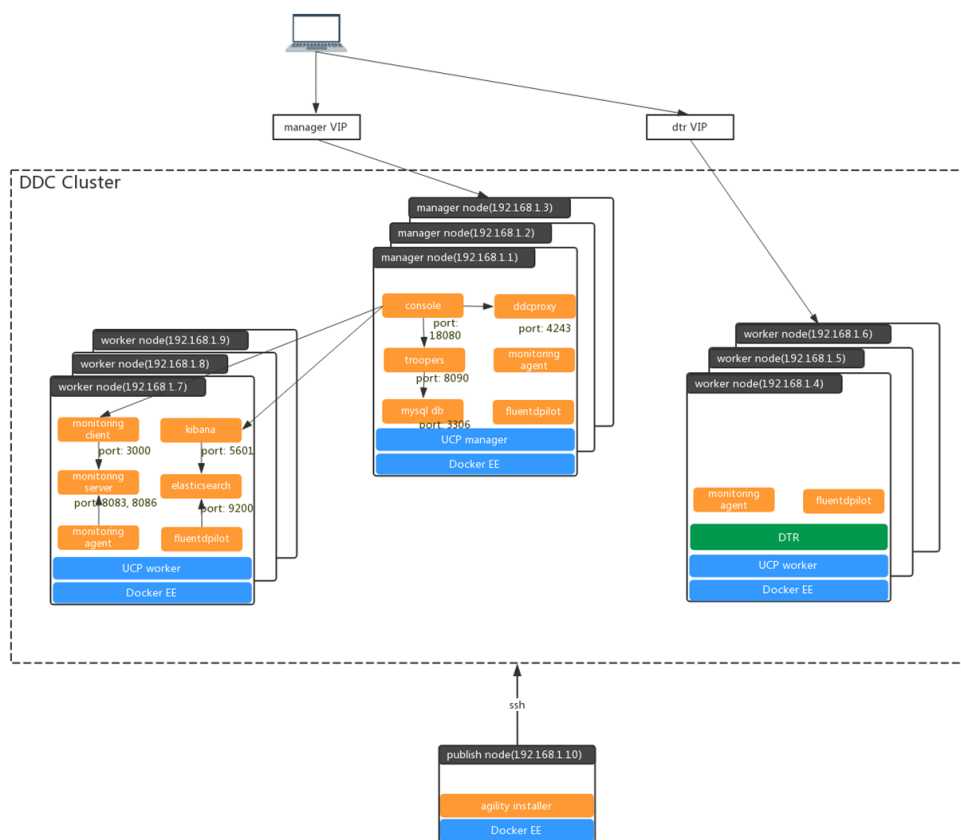
图 5-1: 架构图
