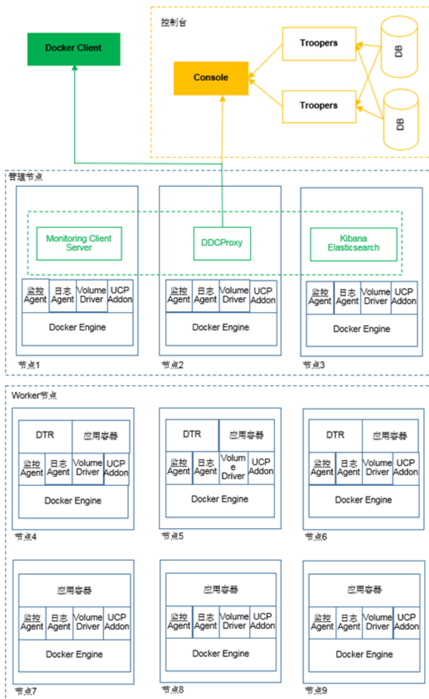
图 5-2: 控制台架构
