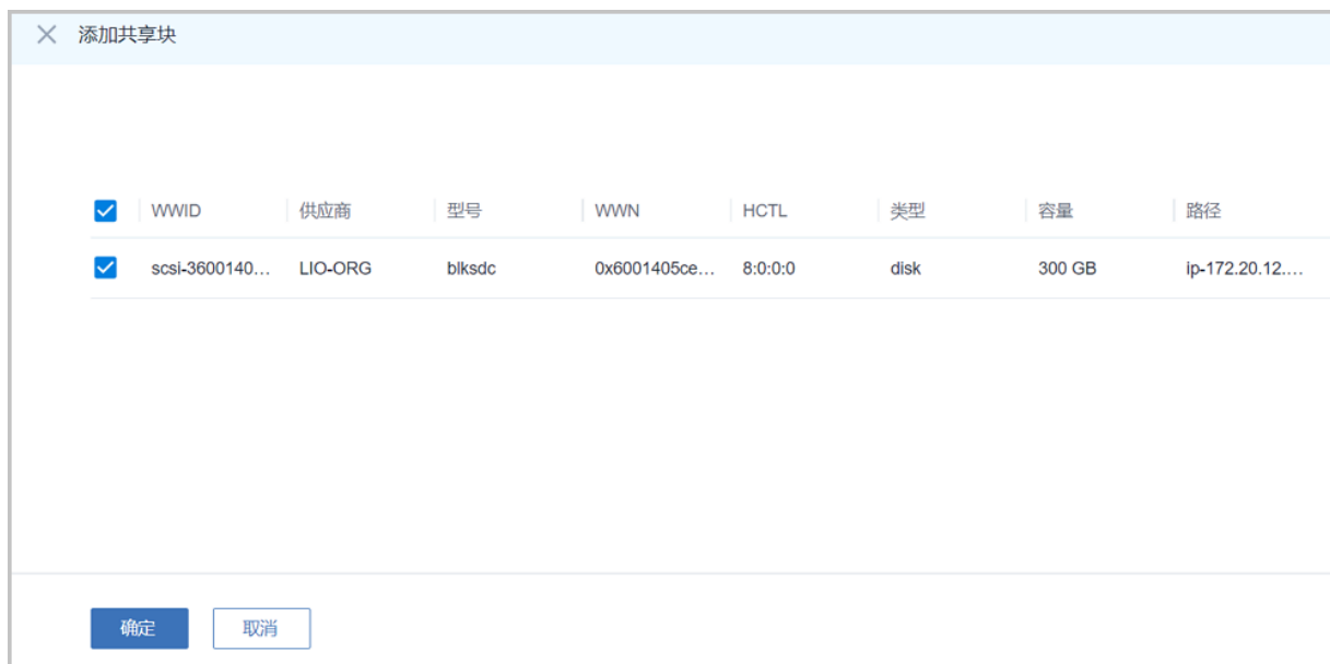
图 4-1: 添加共享块
