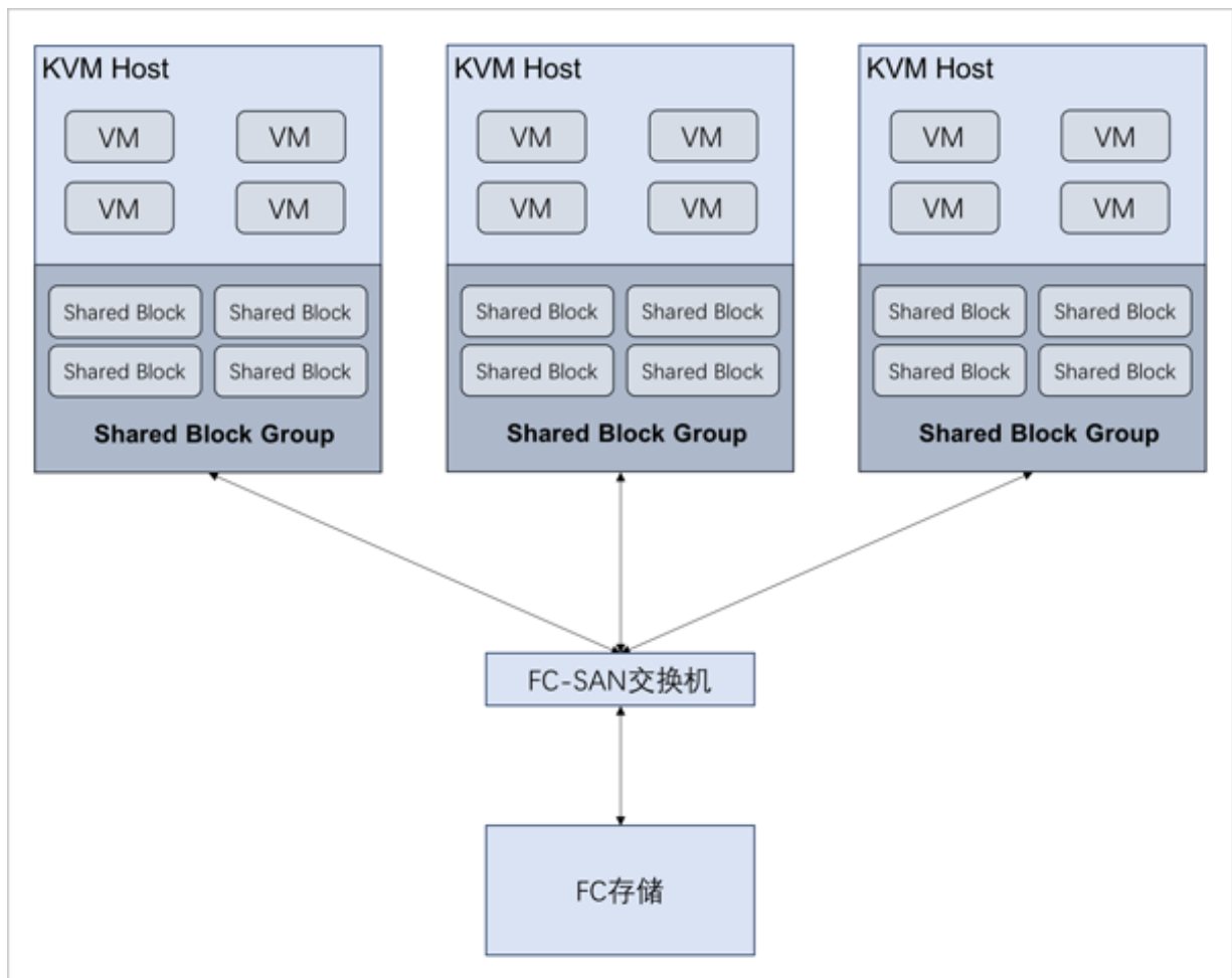
图 2-1: Shared Block与FC存储网络拓扑图
