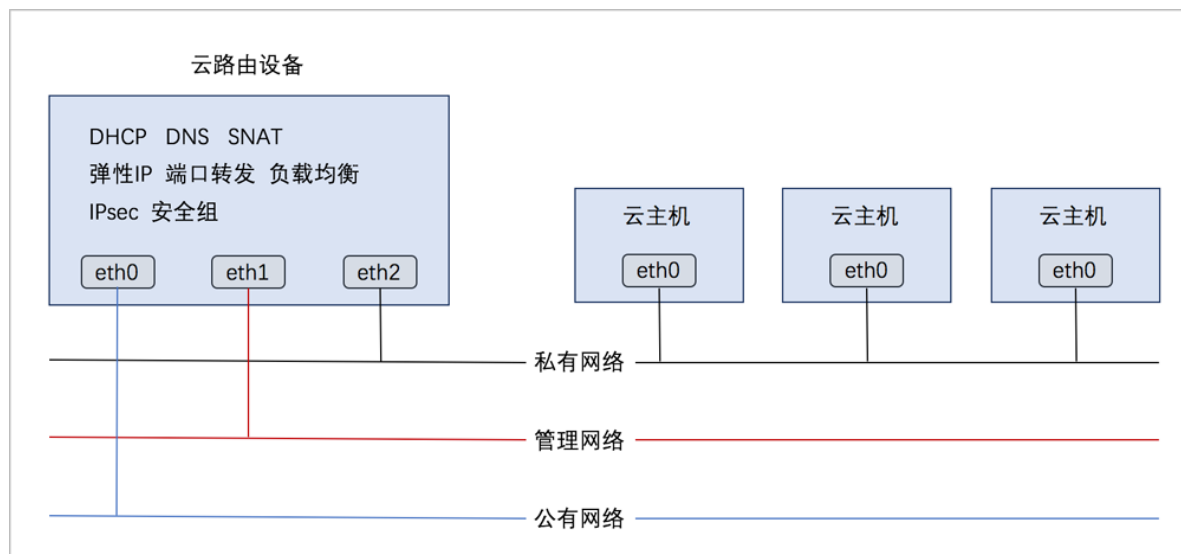
图 2-13: 部署方式-2
