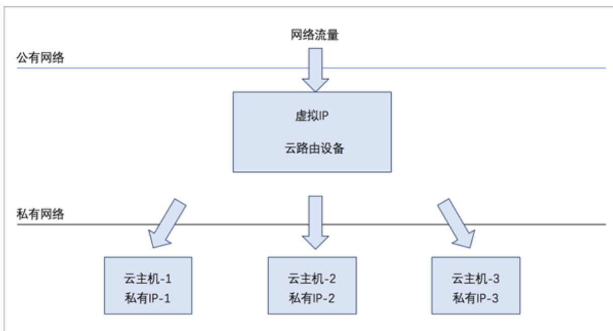
图 2-15: 虚拟IP-负载均衡
