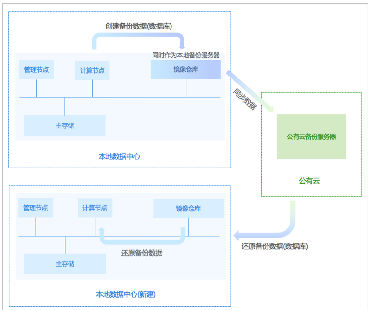
图 2-29: 公共云灾备场景2
