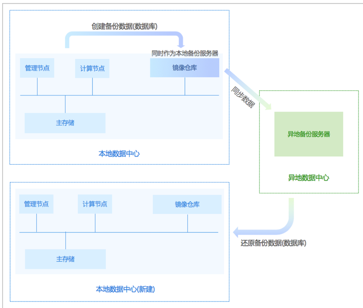
图 2-27: 异地灾备场景2
