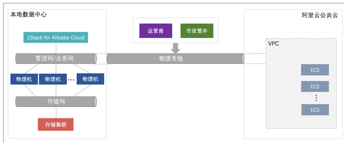
图 2-36: 基于物理专线部署
