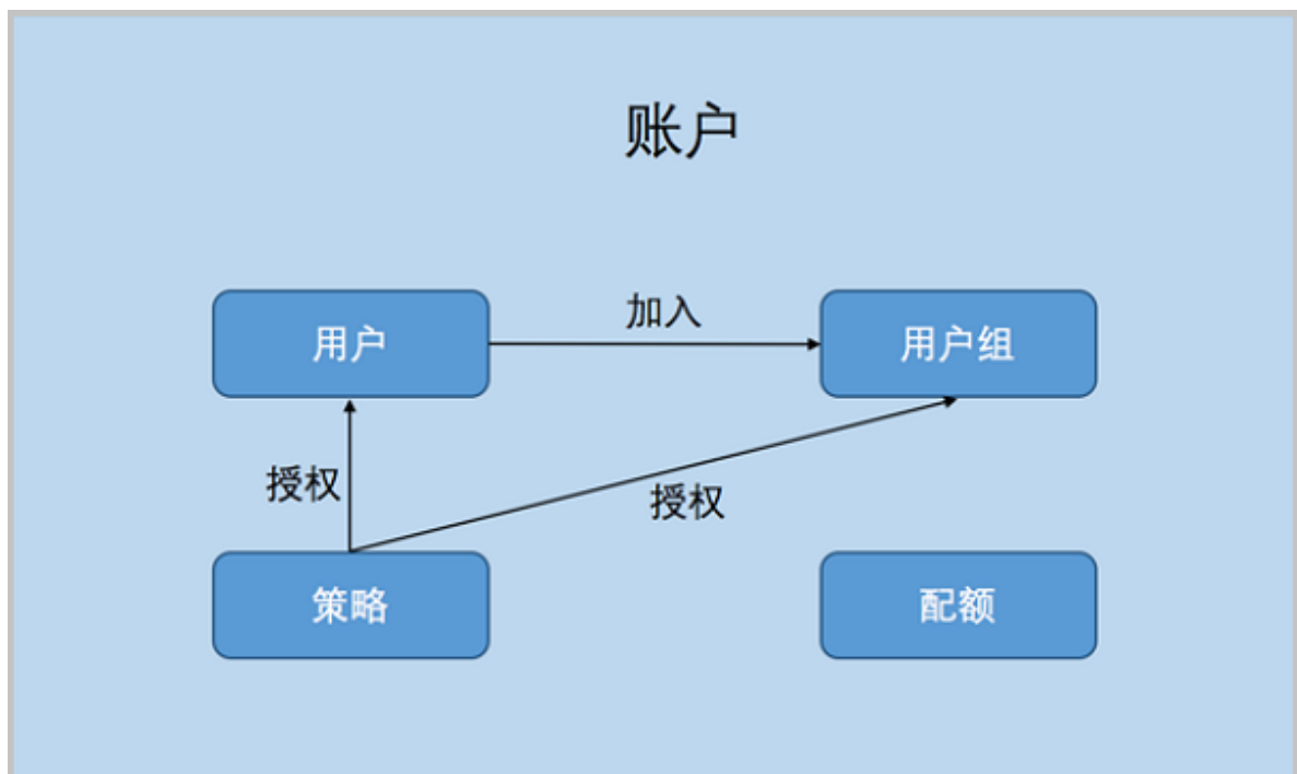
图 2-34: 用户管理系统
