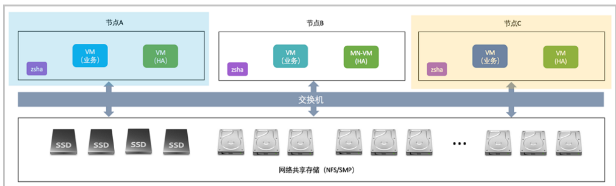
图 2-14: 基于NFS/SMP共享文件系统的高可用集群 经典三节点示例图
