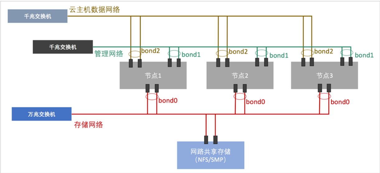
图 1-3: 基于NFS/SMP共享文件系统高可用的三节点网络拓扑
