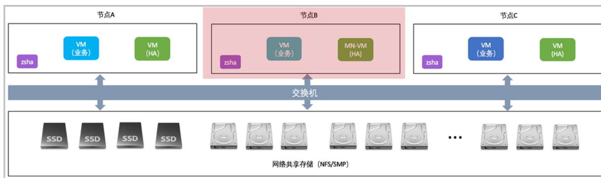
图 2-3: 基于NFS/SMP共享文件系统的高可用集群 经典三节点示例图
