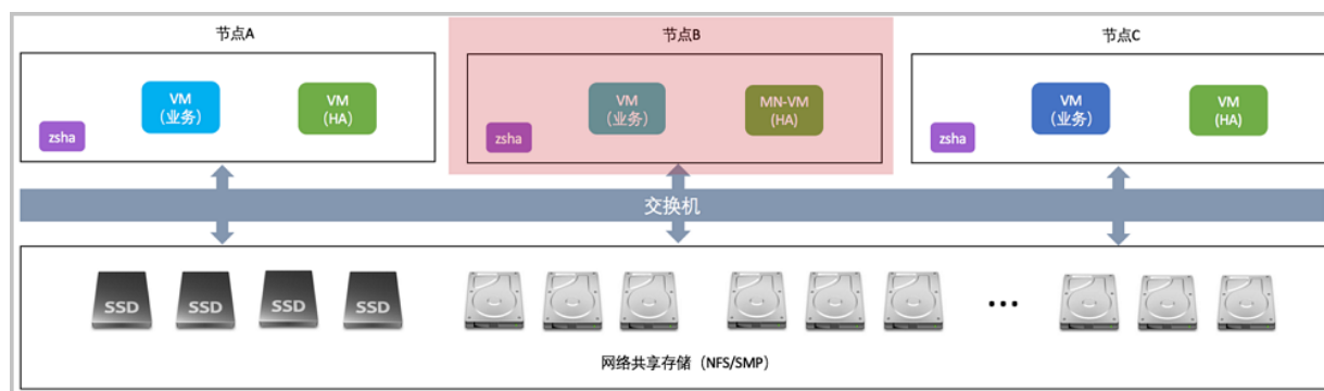
图 2-16: 基于NFS/SMP共享文件系统的高可用集群 经典三节点示例图
