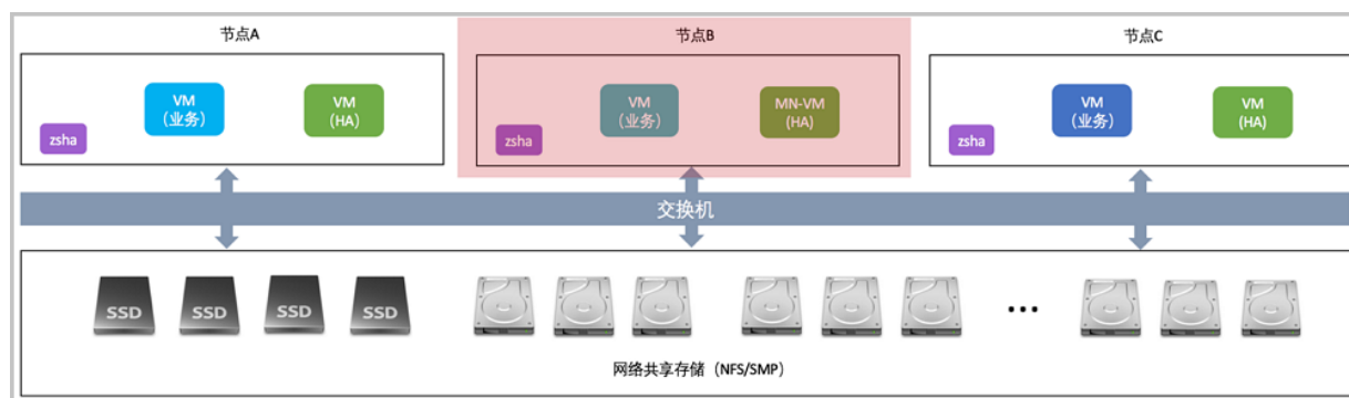
图 2-12: 基于NFS/SMP共享文件系统的高可用集群 经典三节点示例图
