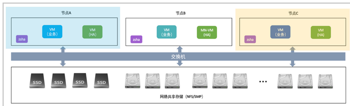
图 2-1: 基于NFS/SMP共享文件系统的高可用集群 经典三节点示例图
