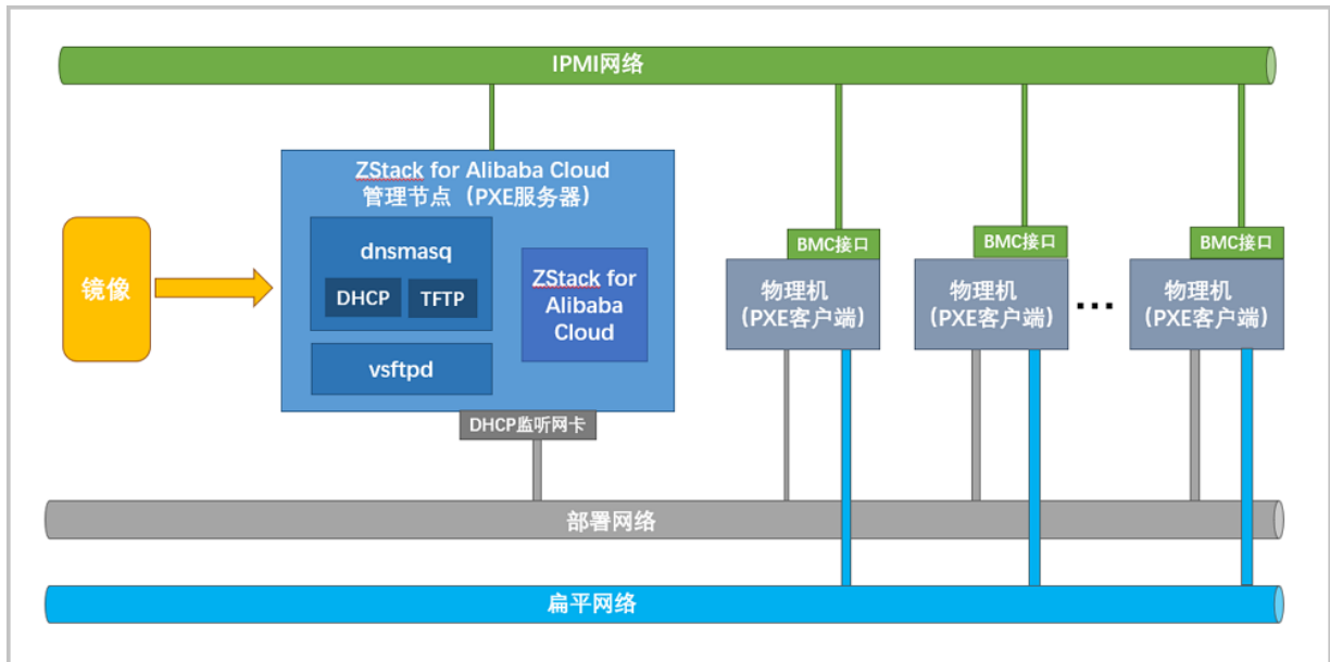
图 2-22: 裸金属管理原理图
