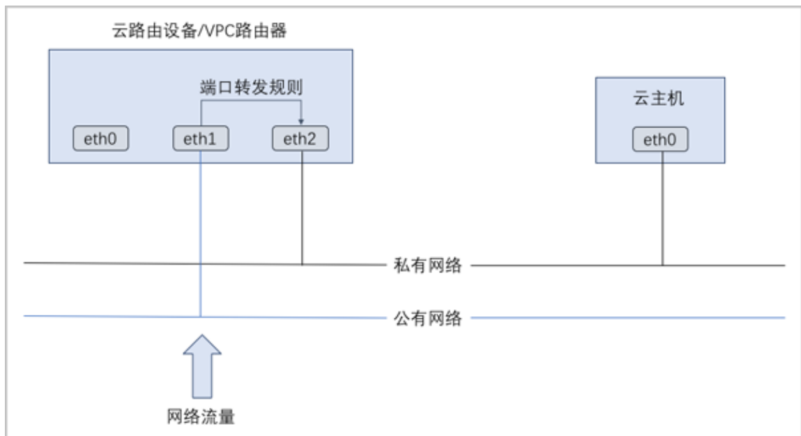
图 2-18: 端口转发
