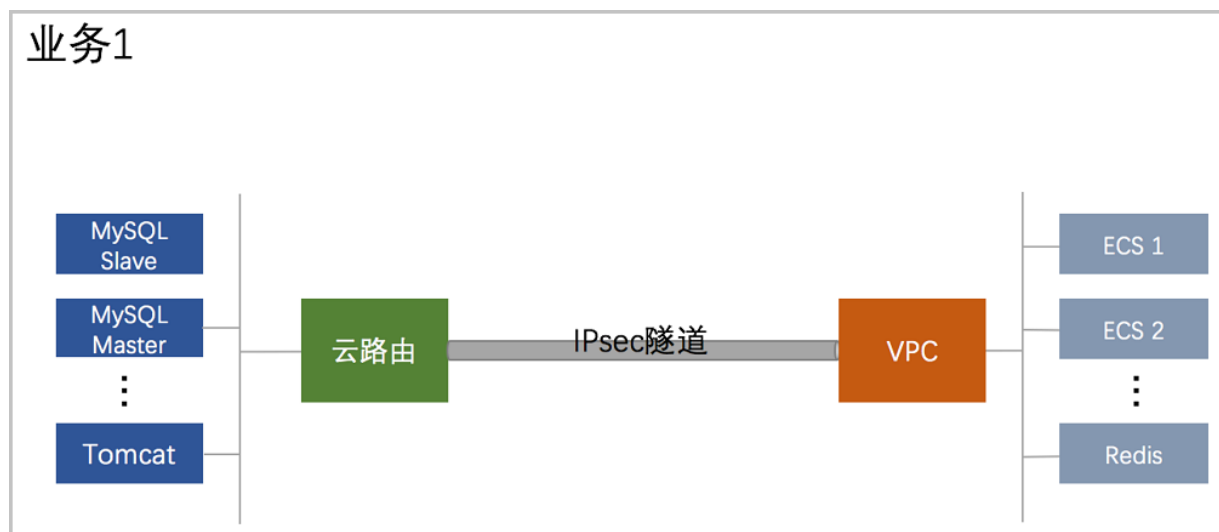
图 2-39: IPsec隧道
