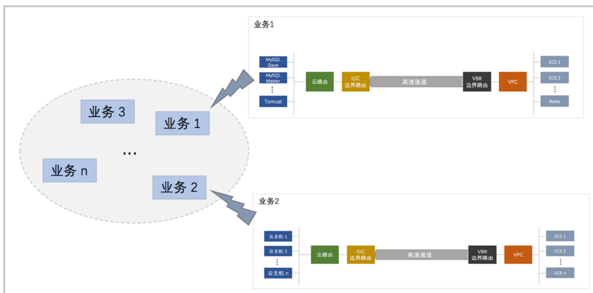
图 2-42: 资源管理
