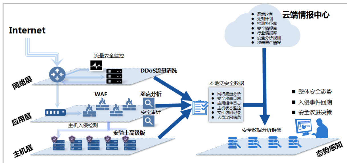
图 16-2: 云盾高级版产品结构图
