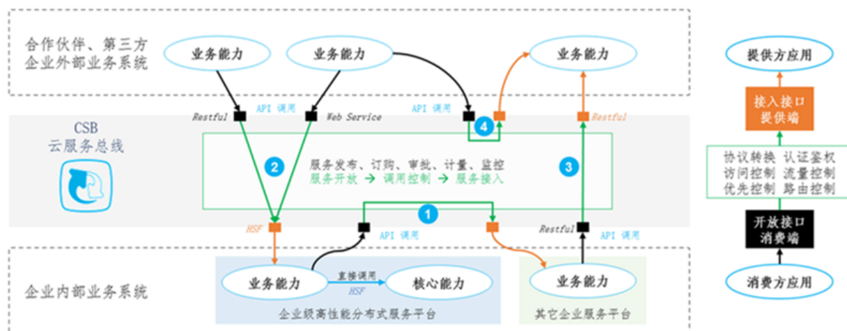
图 22-2: CSB功能示意图
