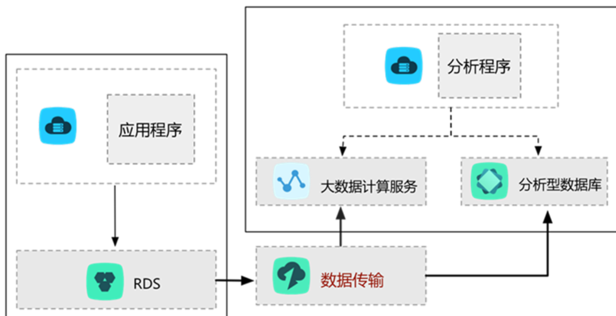
图 13-9: 数据实时分析
