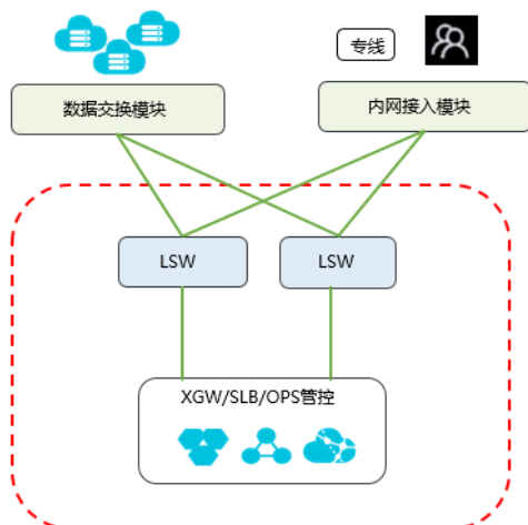
图 3-3: 综合服务模块
