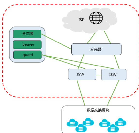
图 3-5: 外网接入模块
