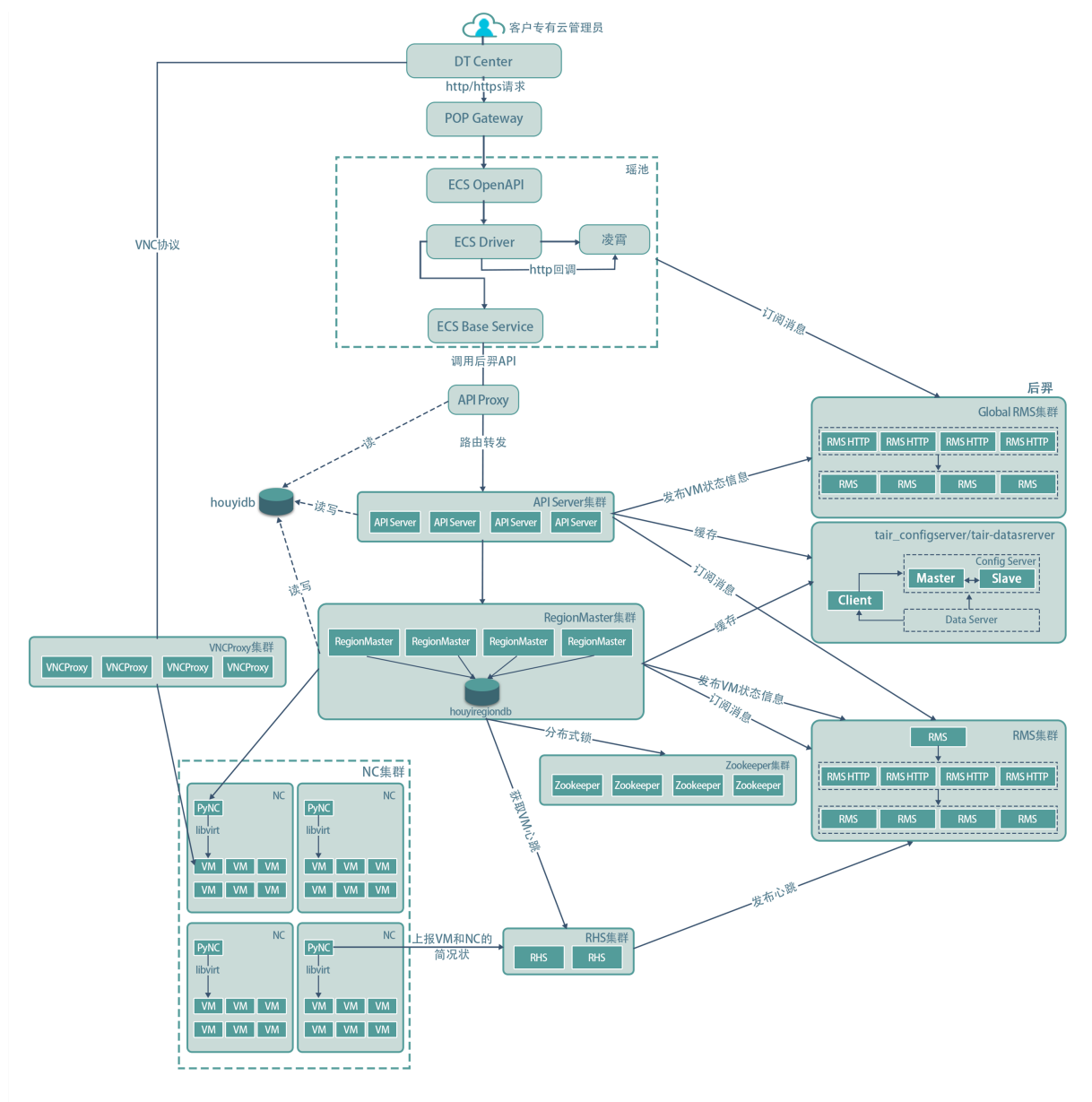
图 7-2: ECS架构图
