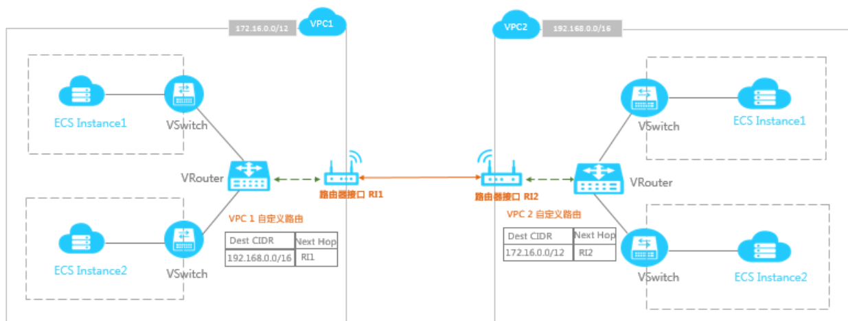
图 15-5: VPC互通
