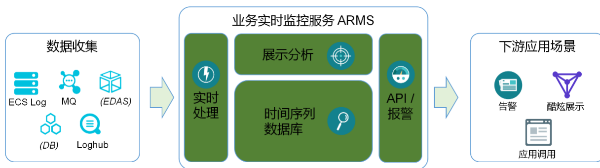
图 21-1: ARMS示意图
