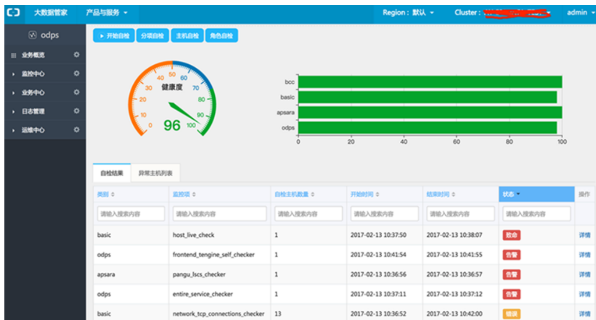
图 28-4: 业务自检图
