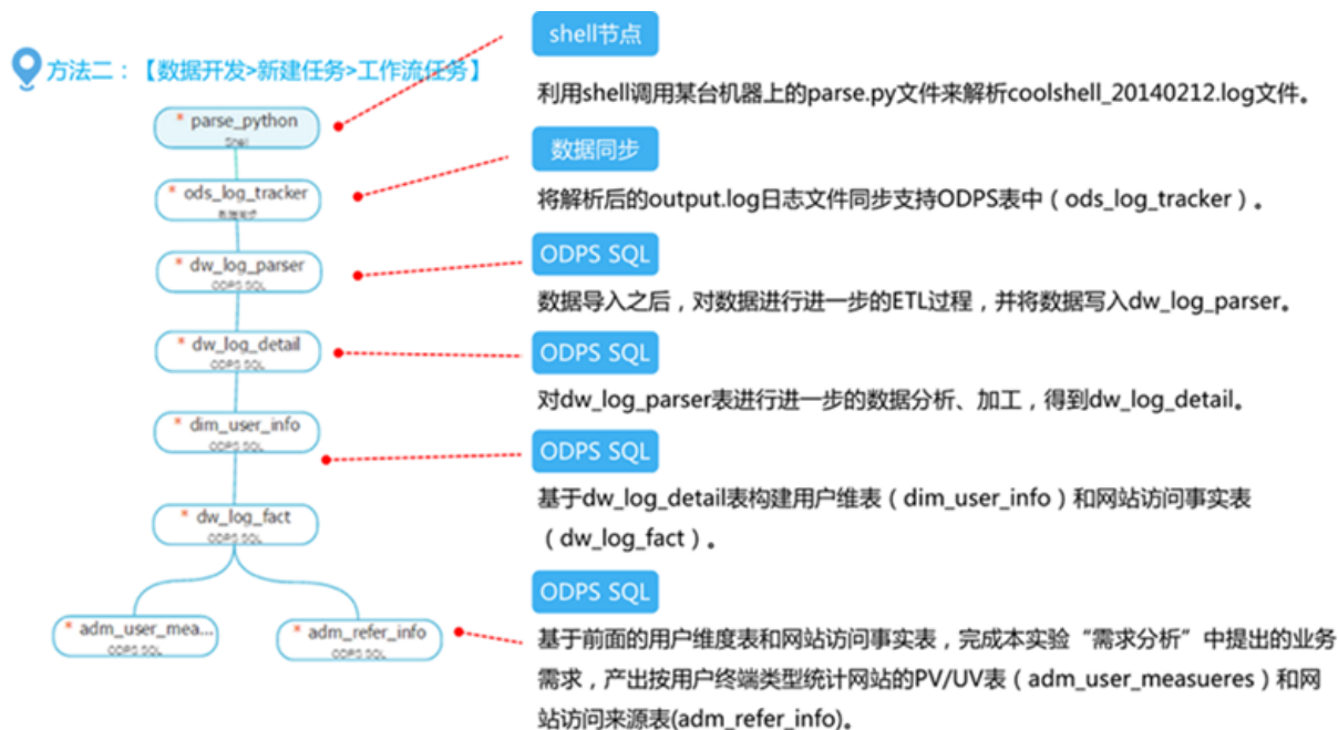
图 24-11: 开发过程
