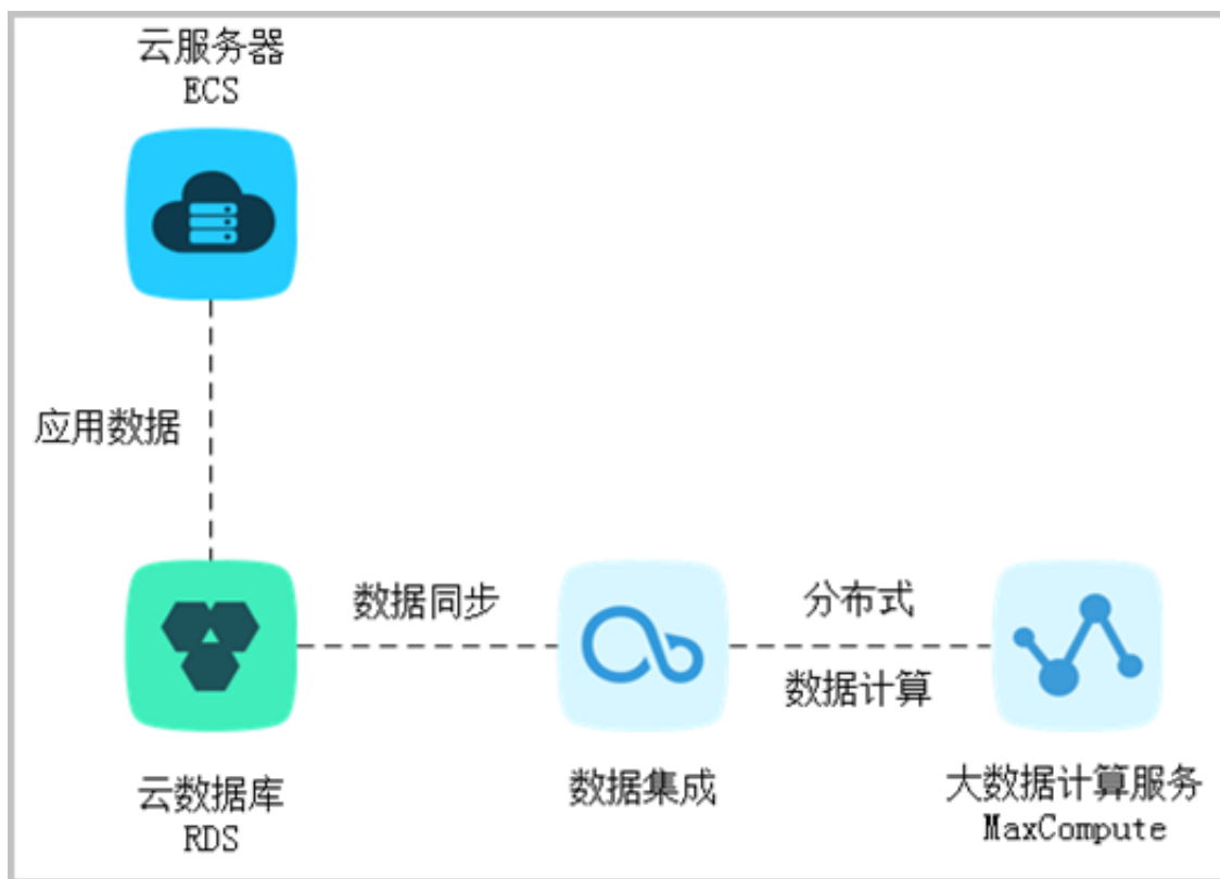
图 11-3: 大数据分析
