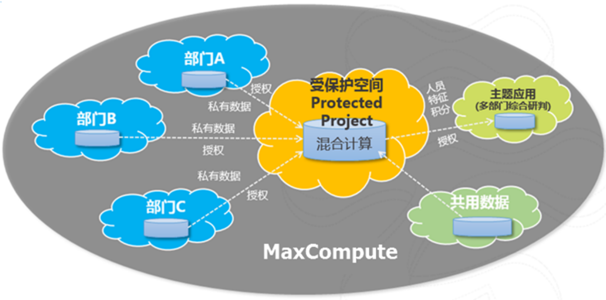
图 23-12: 多租户机制
