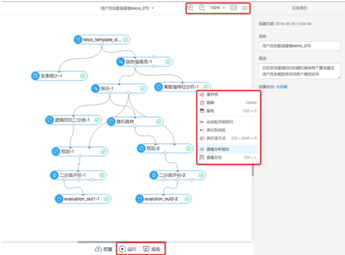
图 31-33: 分析报告
