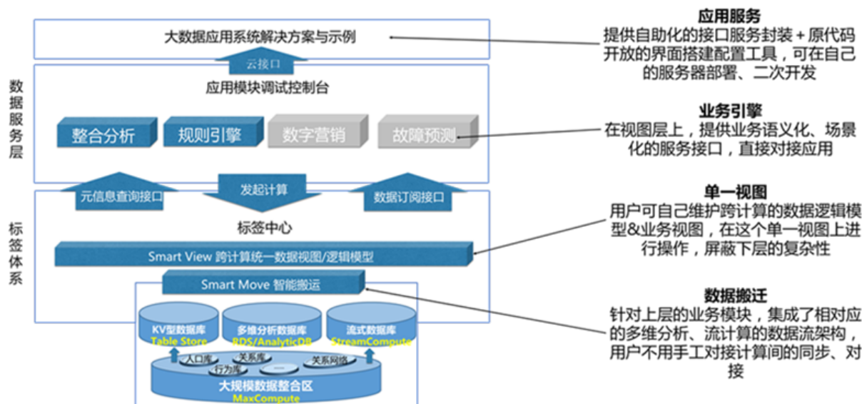
图 27-2: DTBoost架构图
