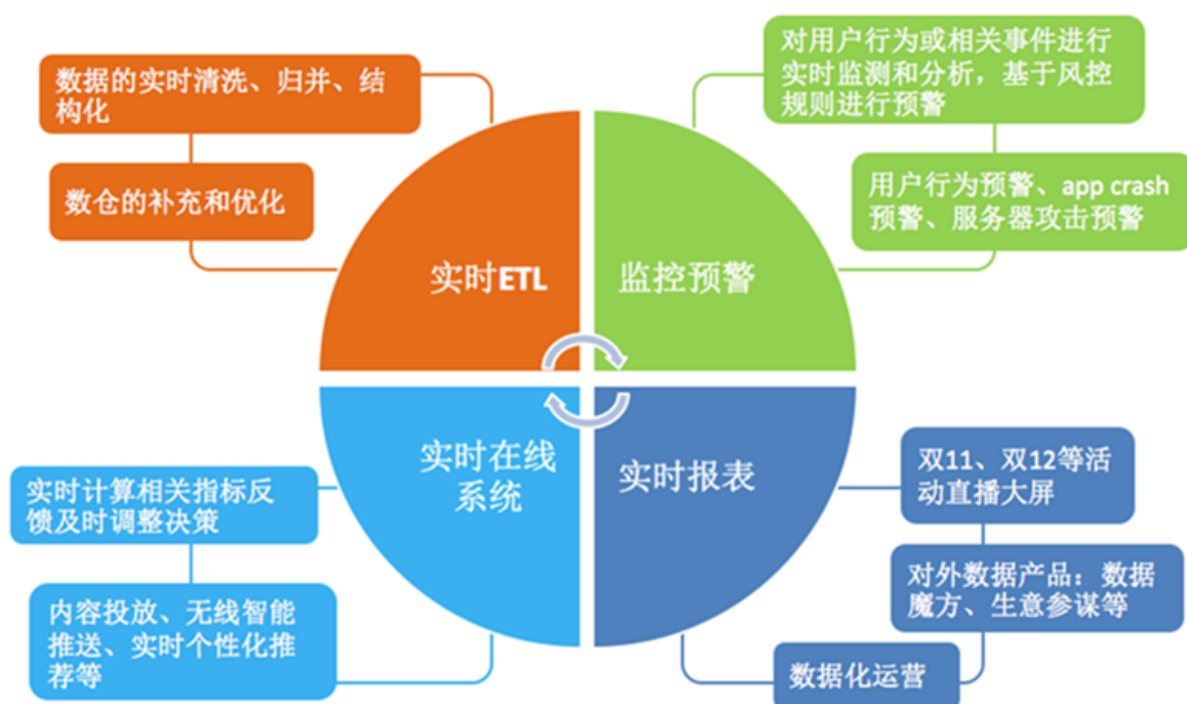
图 26-4: 使用场景
