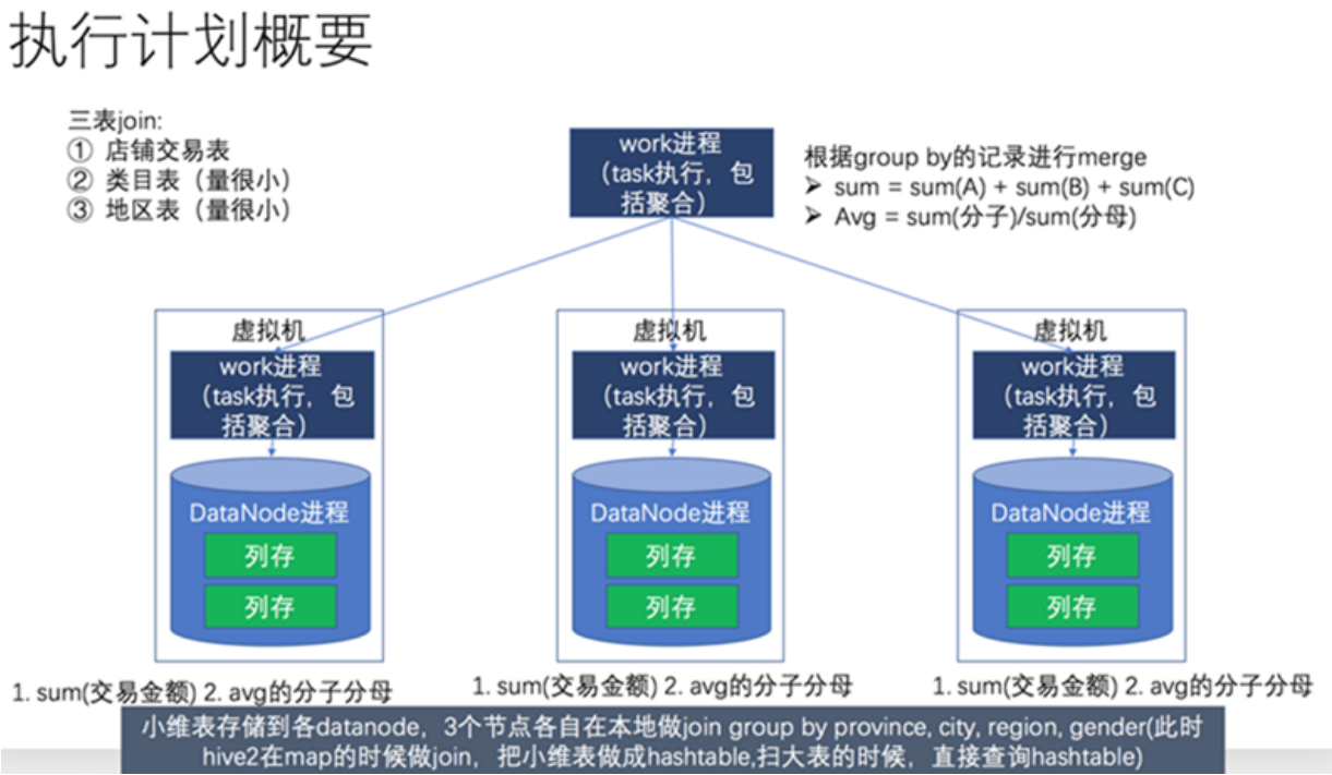
图 31-19: 执行计划
