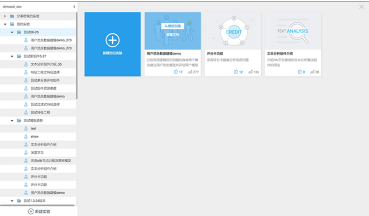
图 31-30: 创建实验
