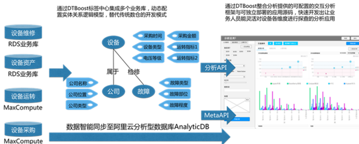
图 27-6: DTBoost应用
