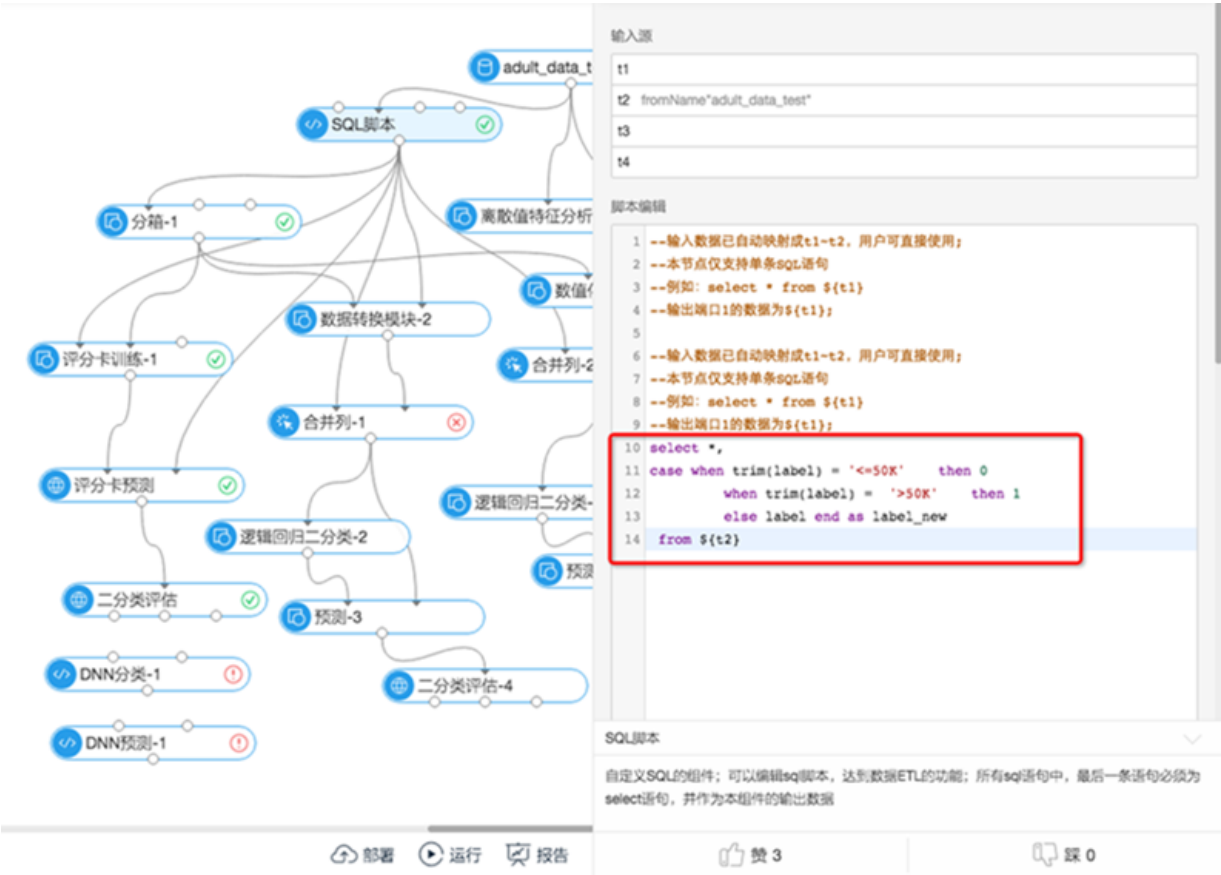
图 31-29: 自定义组件
