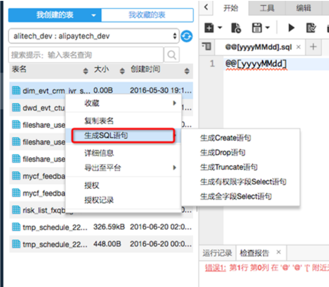
图 31-3: 数据字典
