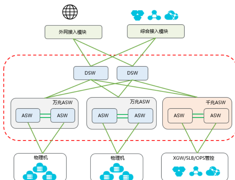
图 3-2: 数据库交换模块
