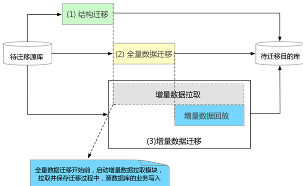
图 13-2: 数据迁移基本原理图
