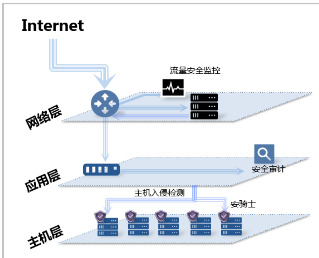
图 16-1: 云盾基础版产品结构图
