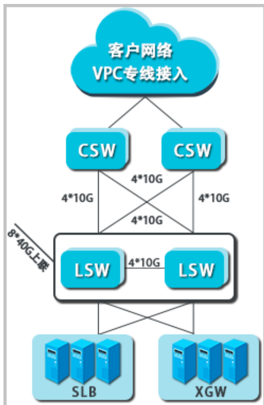
图 3-6: VPC专线接入示意图
