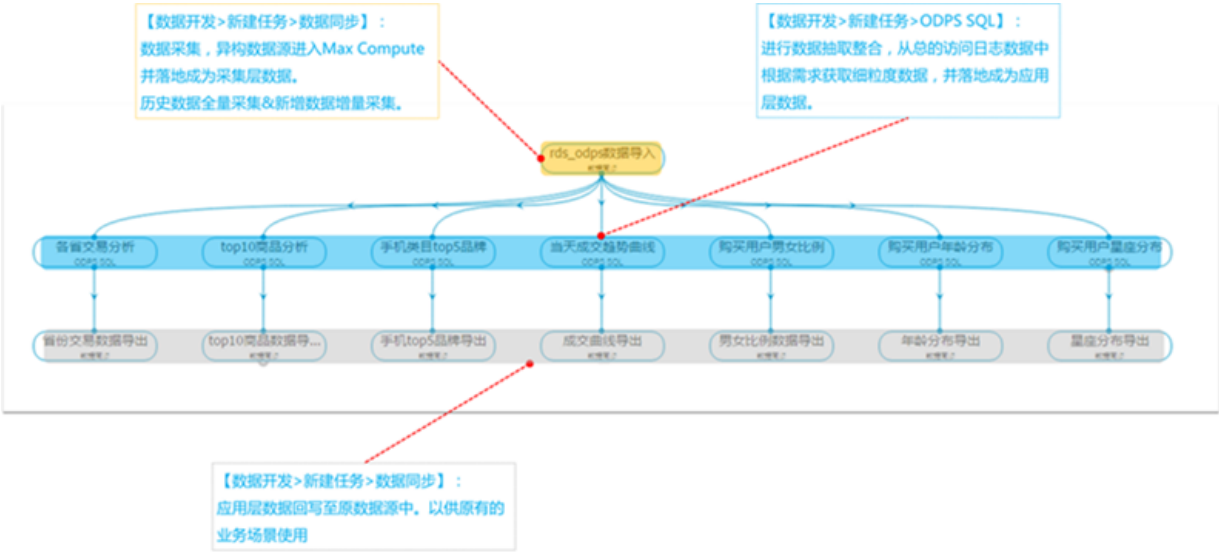
图 24-14: 任务管理
