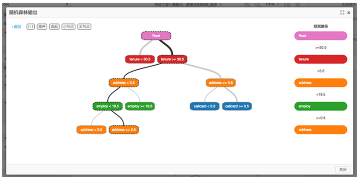
图 31-42: 模型可视化
