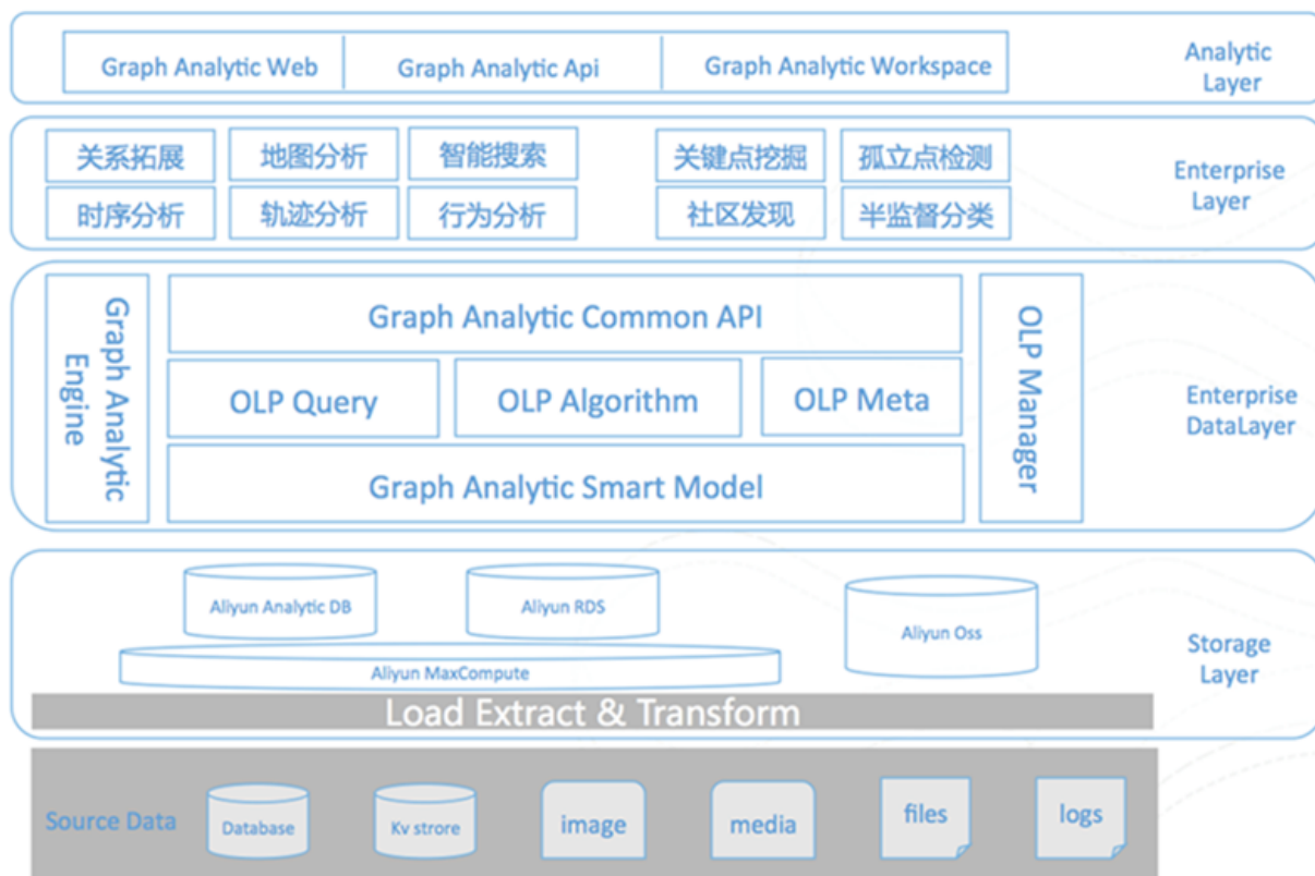
图 30-6: 系统架构
