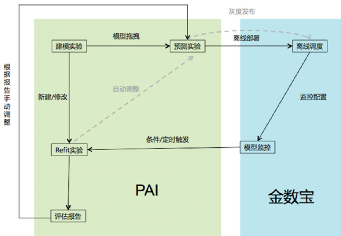
图 31-37: 模型回溯
