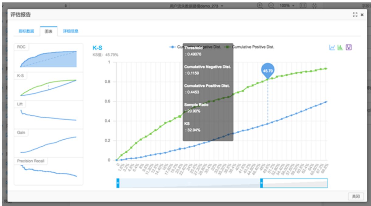
图 31-39: 评估可视化
