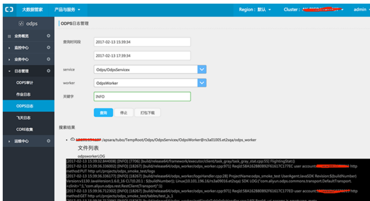
图 28-6: 日志管理图
