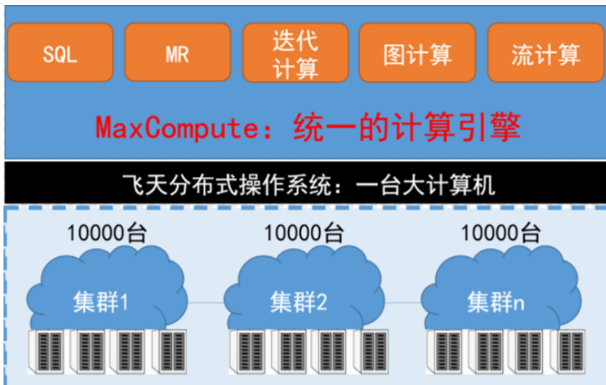
图 23-11: 操作系统
