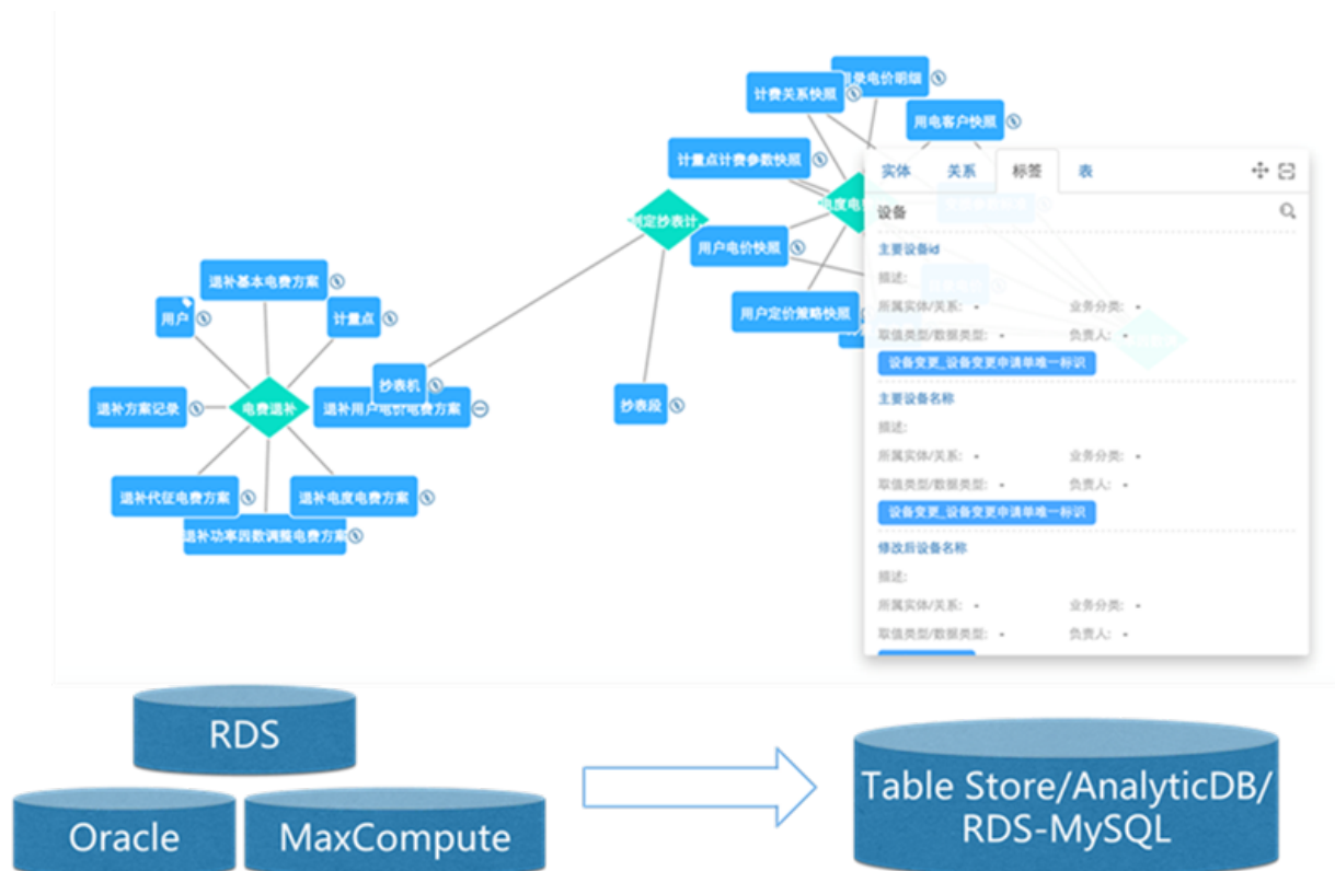
图 27-3: DTBoost功能
