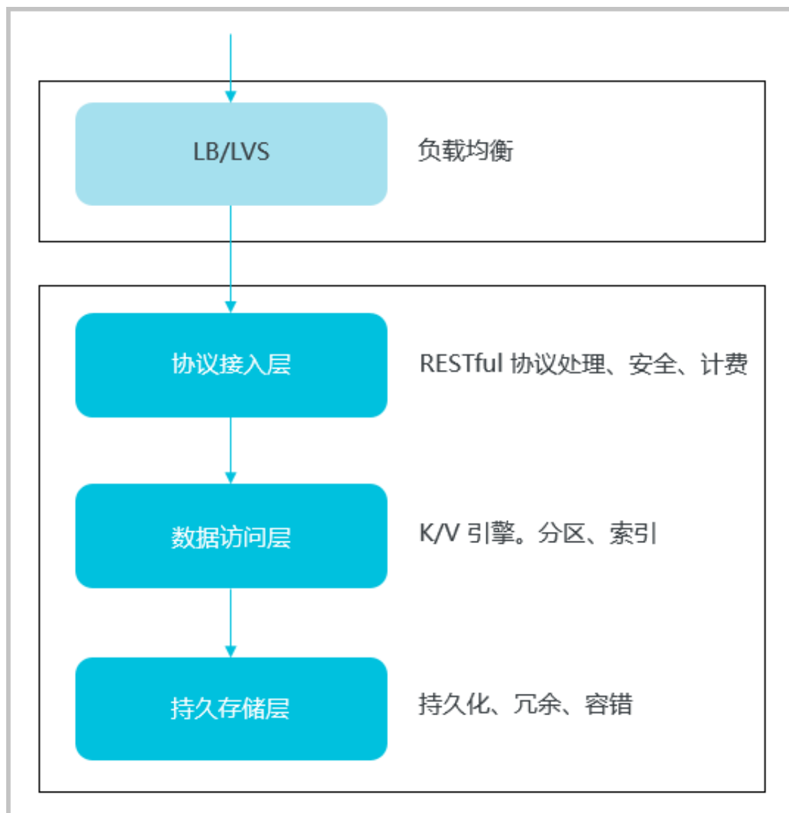
图 9-1: OSS 架构图
