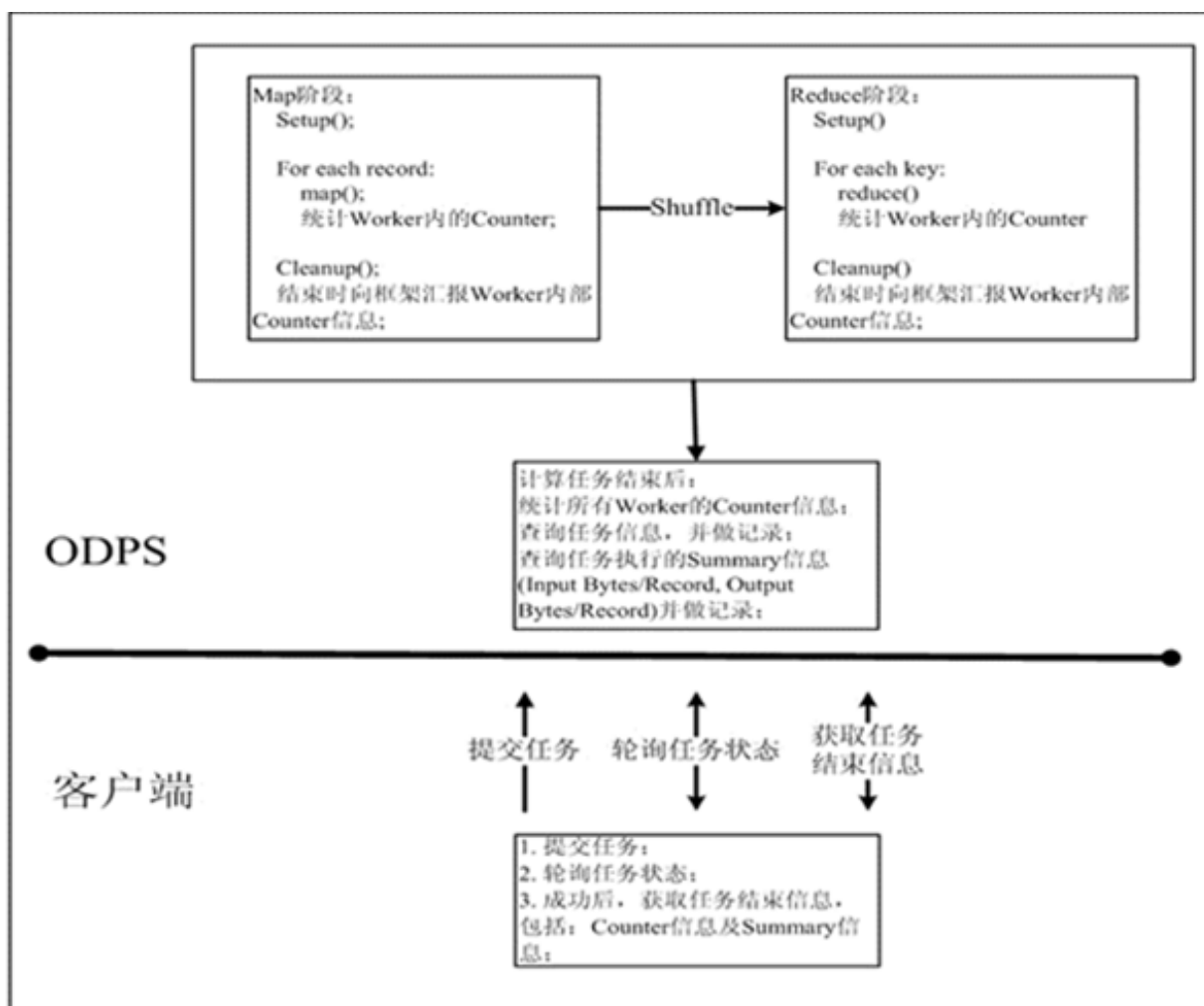
图 23-5: MR过程
