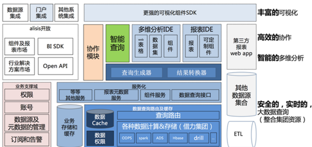
图 31-21: 架构图
