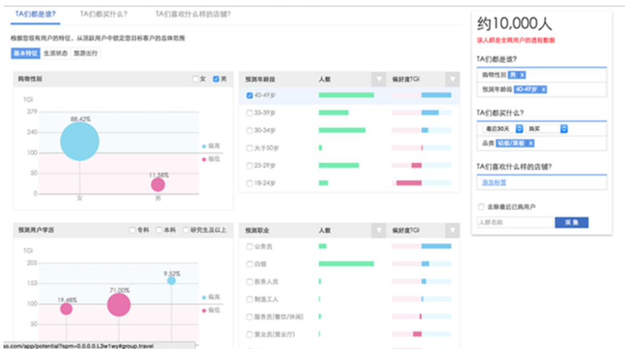
图 27-7: 画像分析
