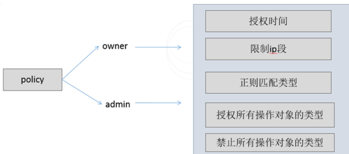
图 23-8: policy授权
