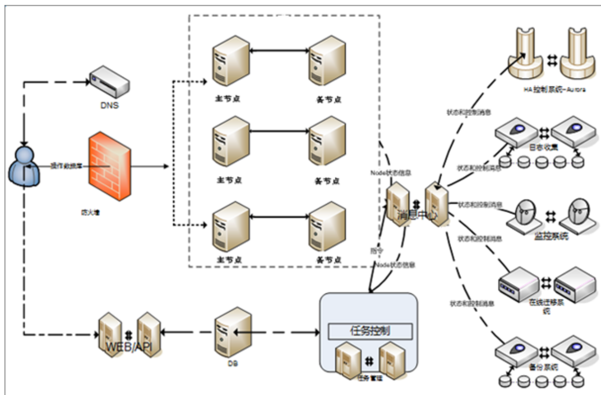
图 12-1: 架构图
