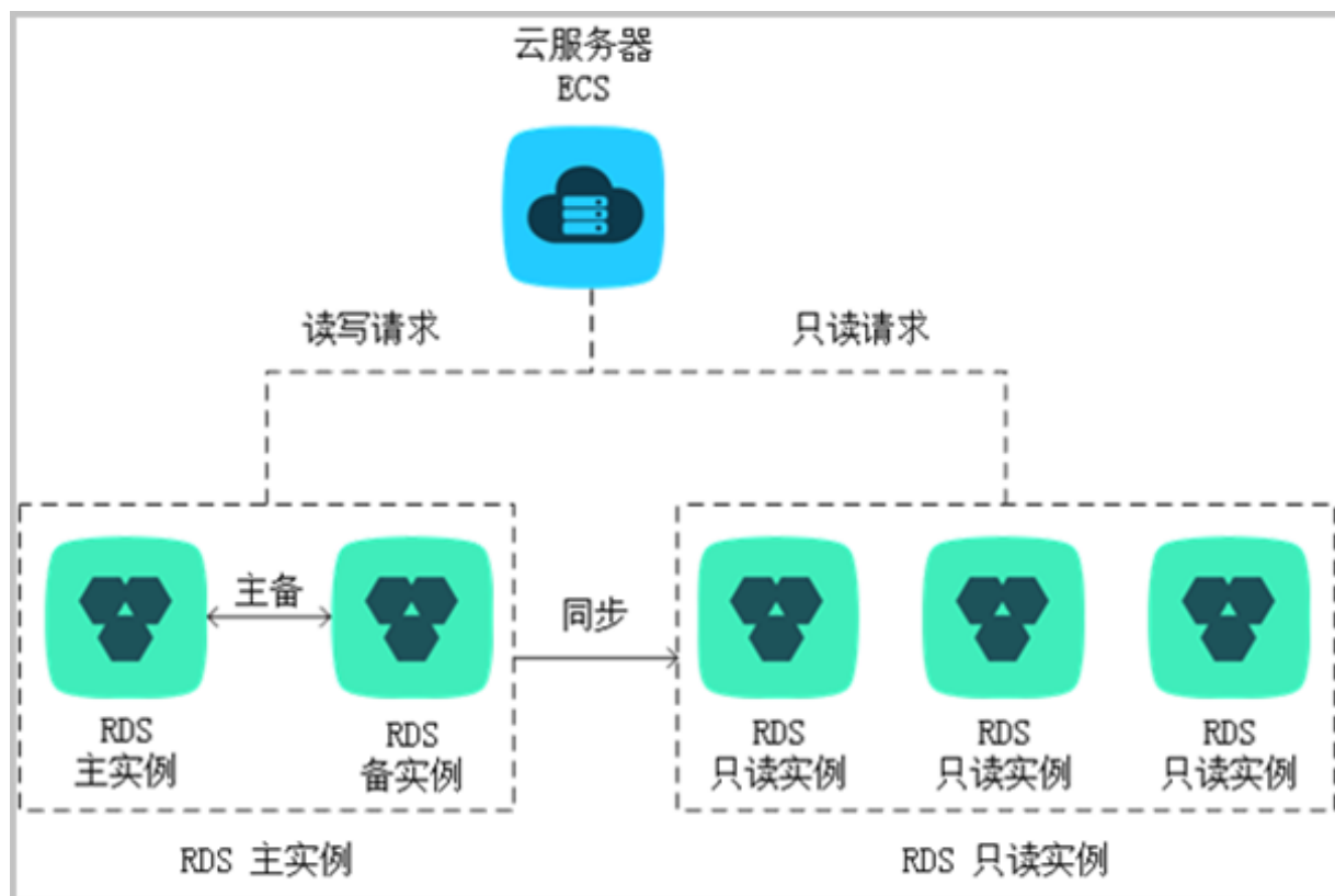
图 11-2: 读写分离
