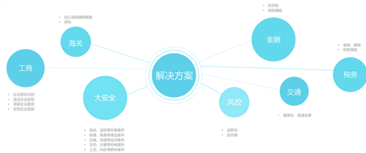
图 30-13: 典型应用
