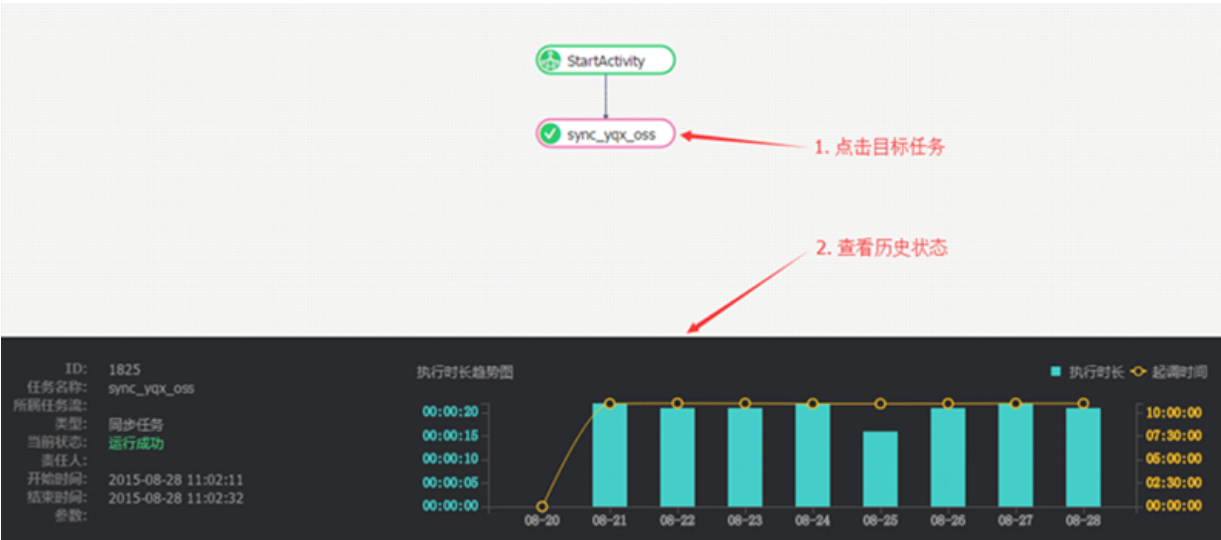
图 31-6: 任务监控
