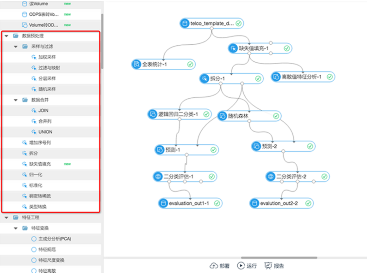
图 31-25: 预处理组件
