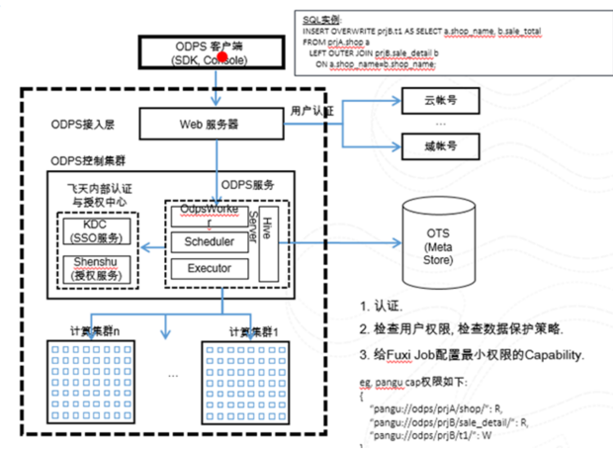
图 23-7: 安全架构
